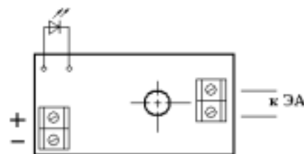
Рис. 3 – Схема подключения «Гарант-12КД» исп. 2
