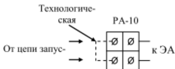
Рис. 2 – Схема подключения «Гарант-12КД» исп. 1
